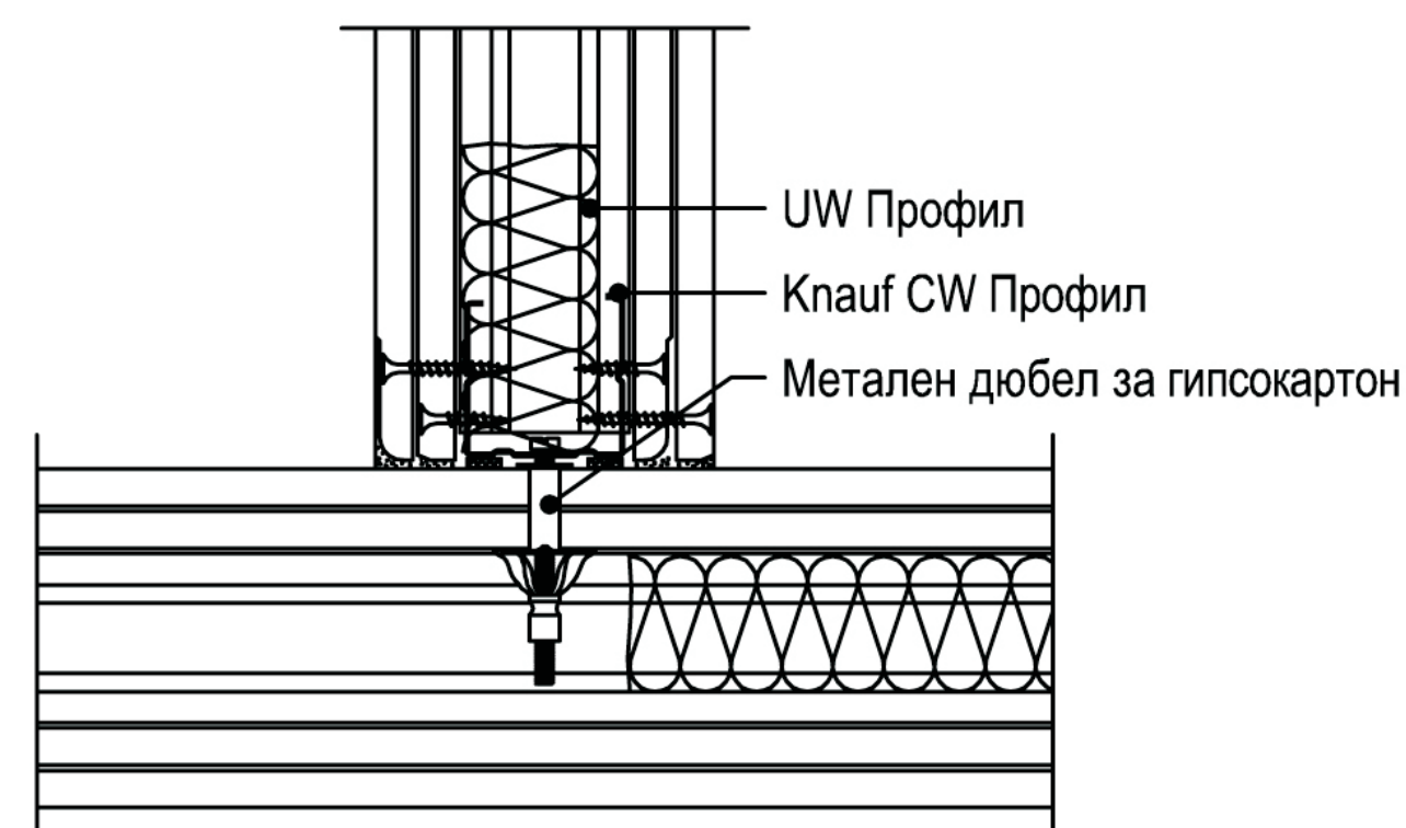
6' Т-образна връзка с дюбел за ГК без профил
