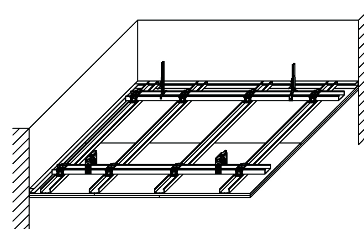
1A Окачване чрез "окачвачи"
