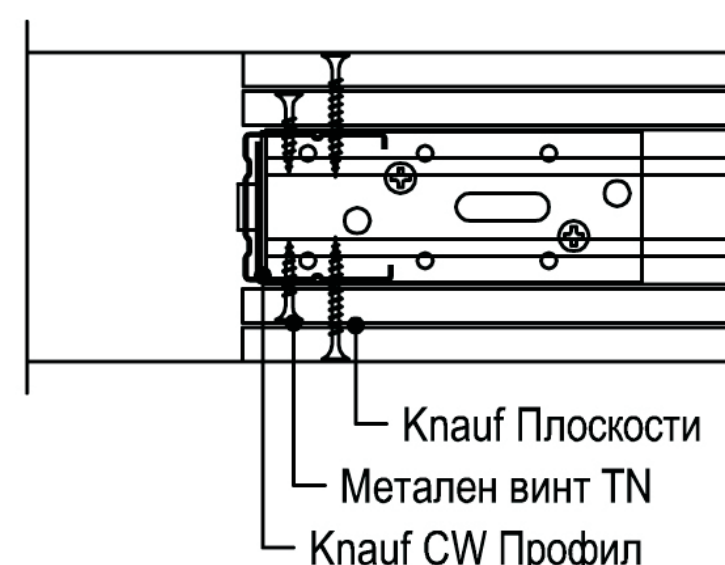
3 Отвор за врата
