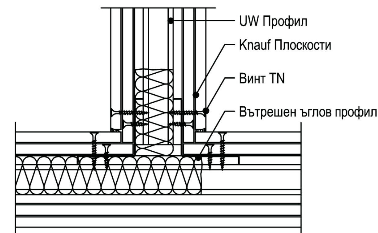
6'' Т-образна връзка с вътрешни ъглови профили
