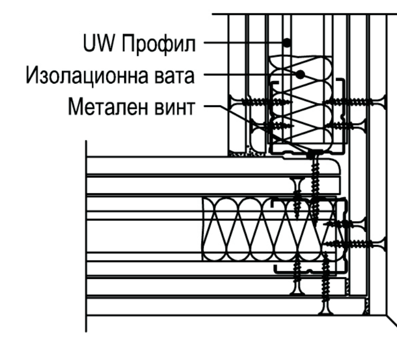
5 Ъглова връзка
