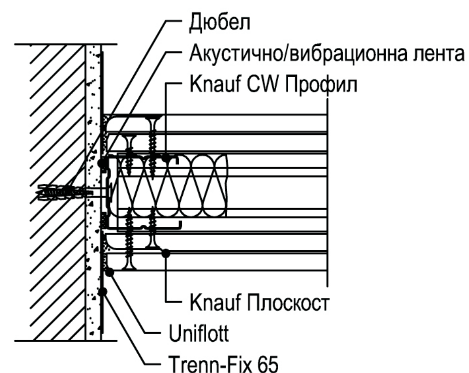
2 Връзка с масивна стена
