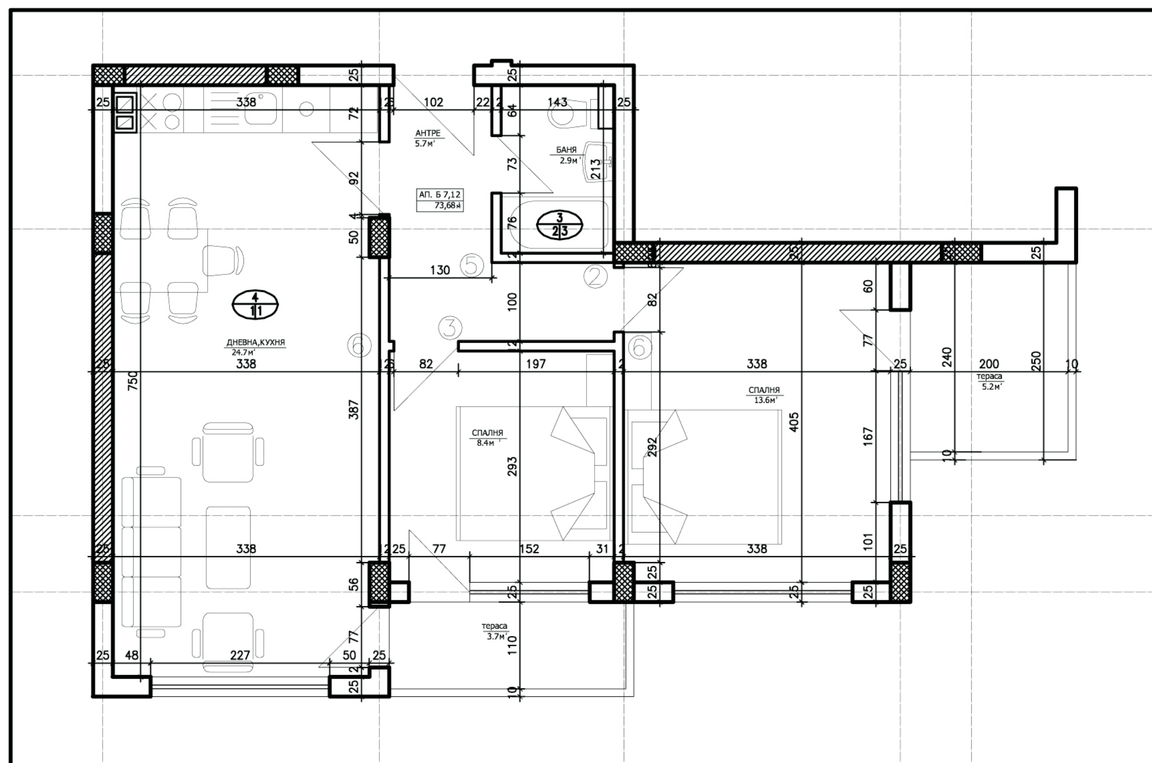
Разпределение на апартамент
