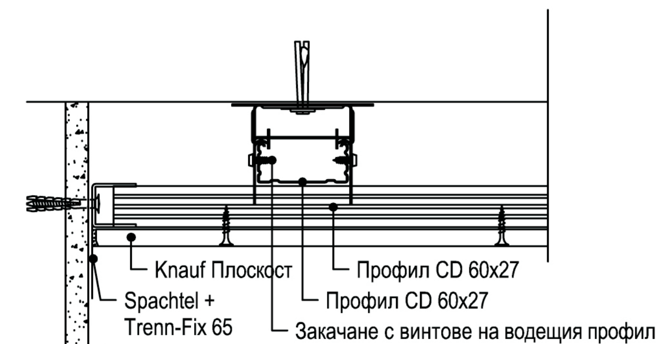
1 Непосредствено окачване за тавана
