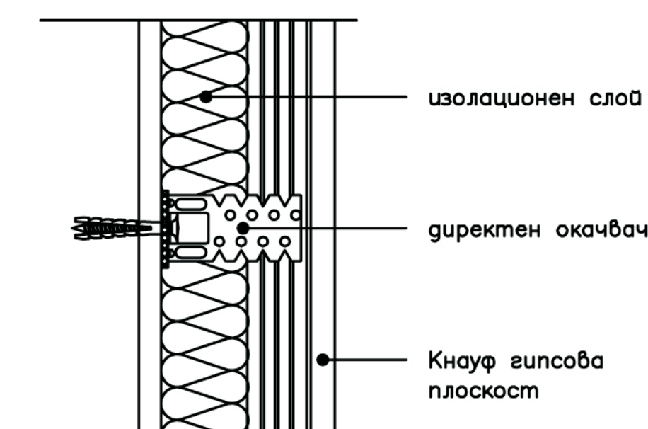
7 Предстенна обшивка
