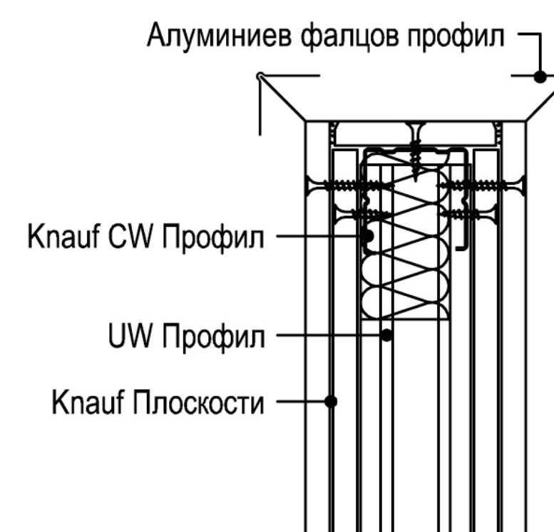
4 Отвор без врата/прозорец
