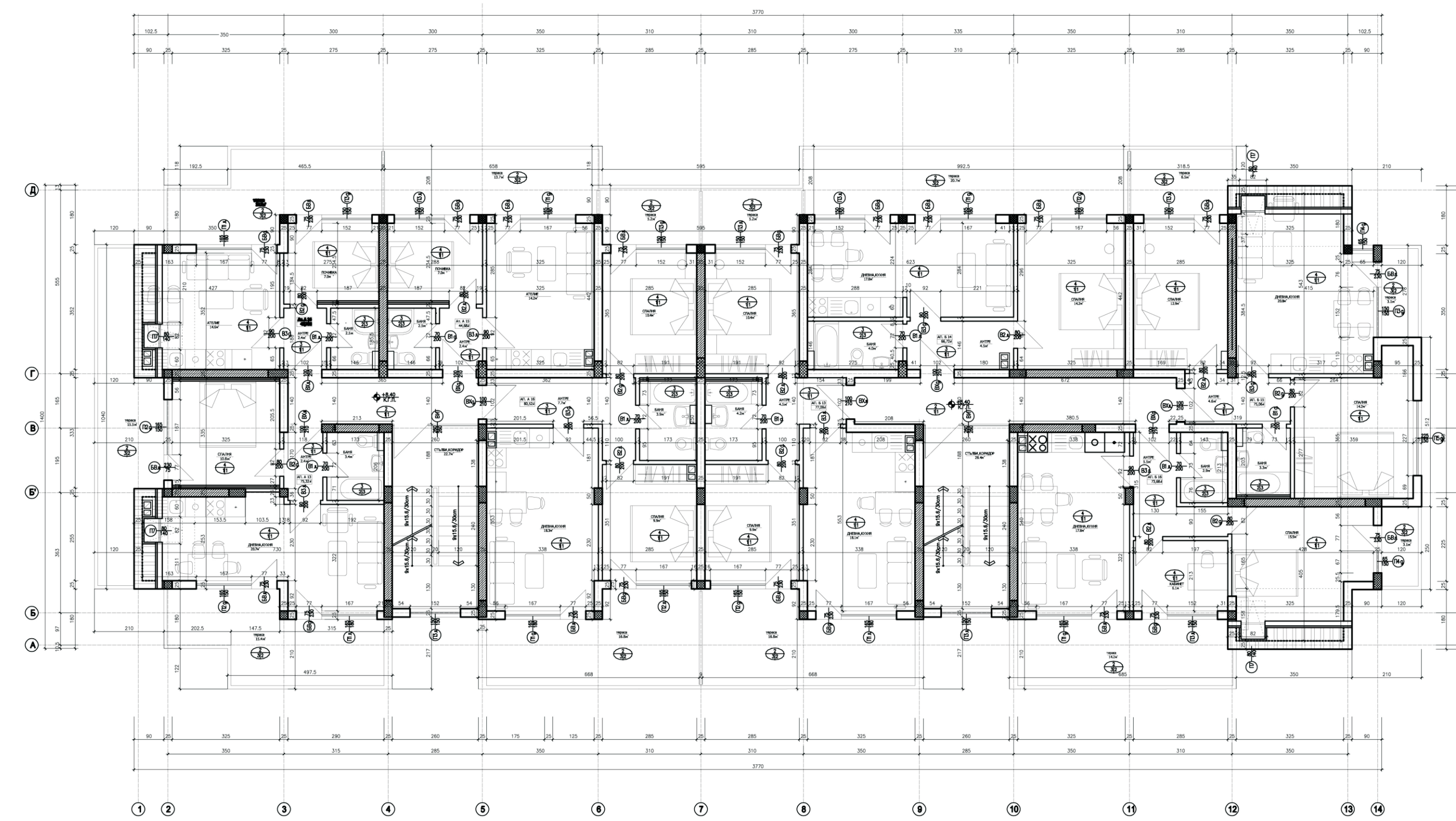
разпределение терасовиден етаж
