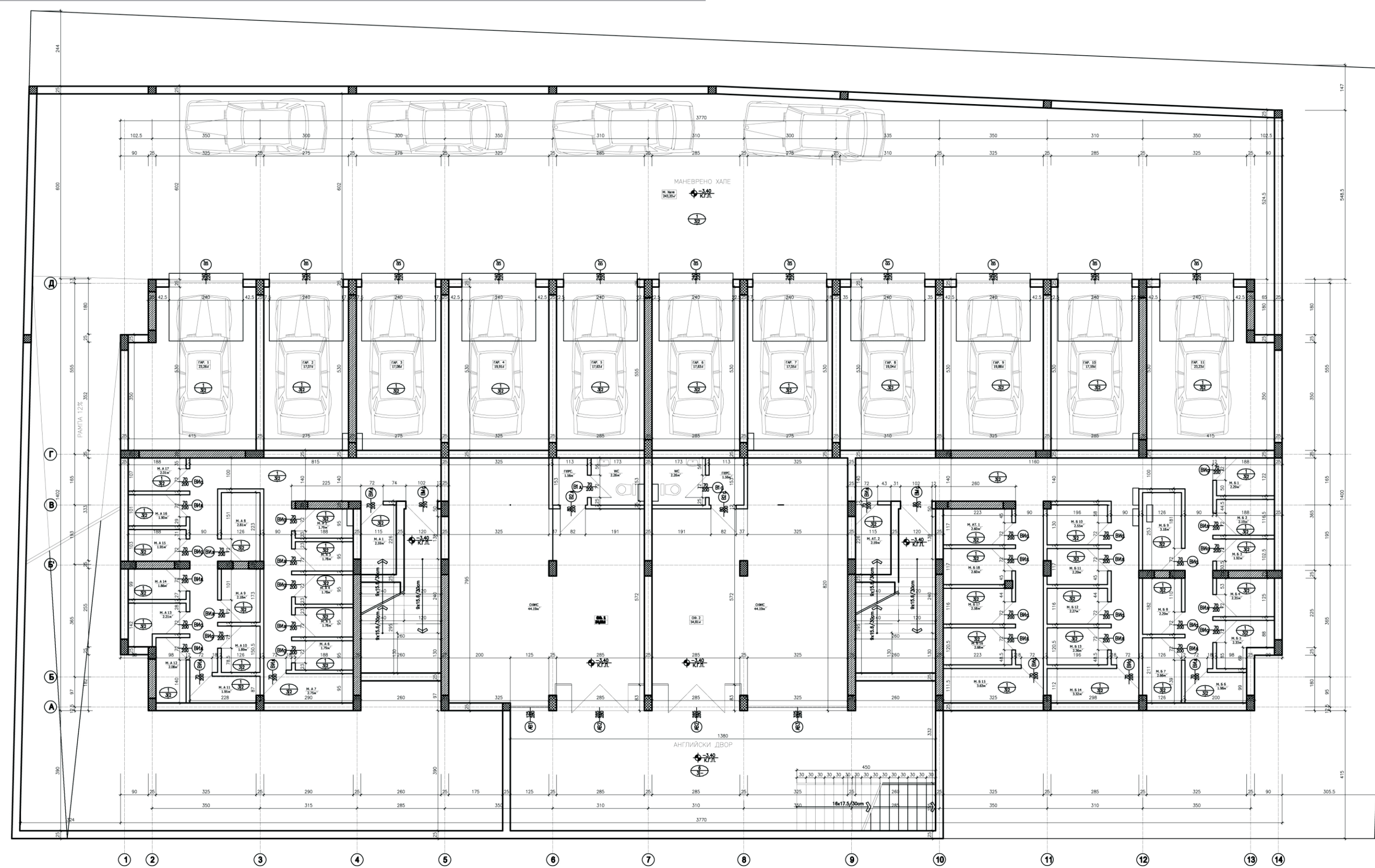
разпределение сутерен
