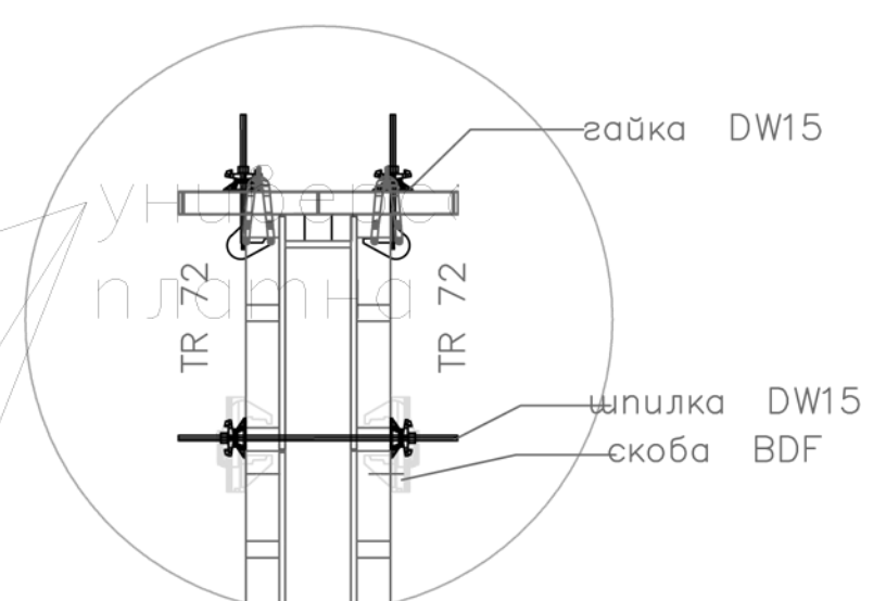
Детайл А
