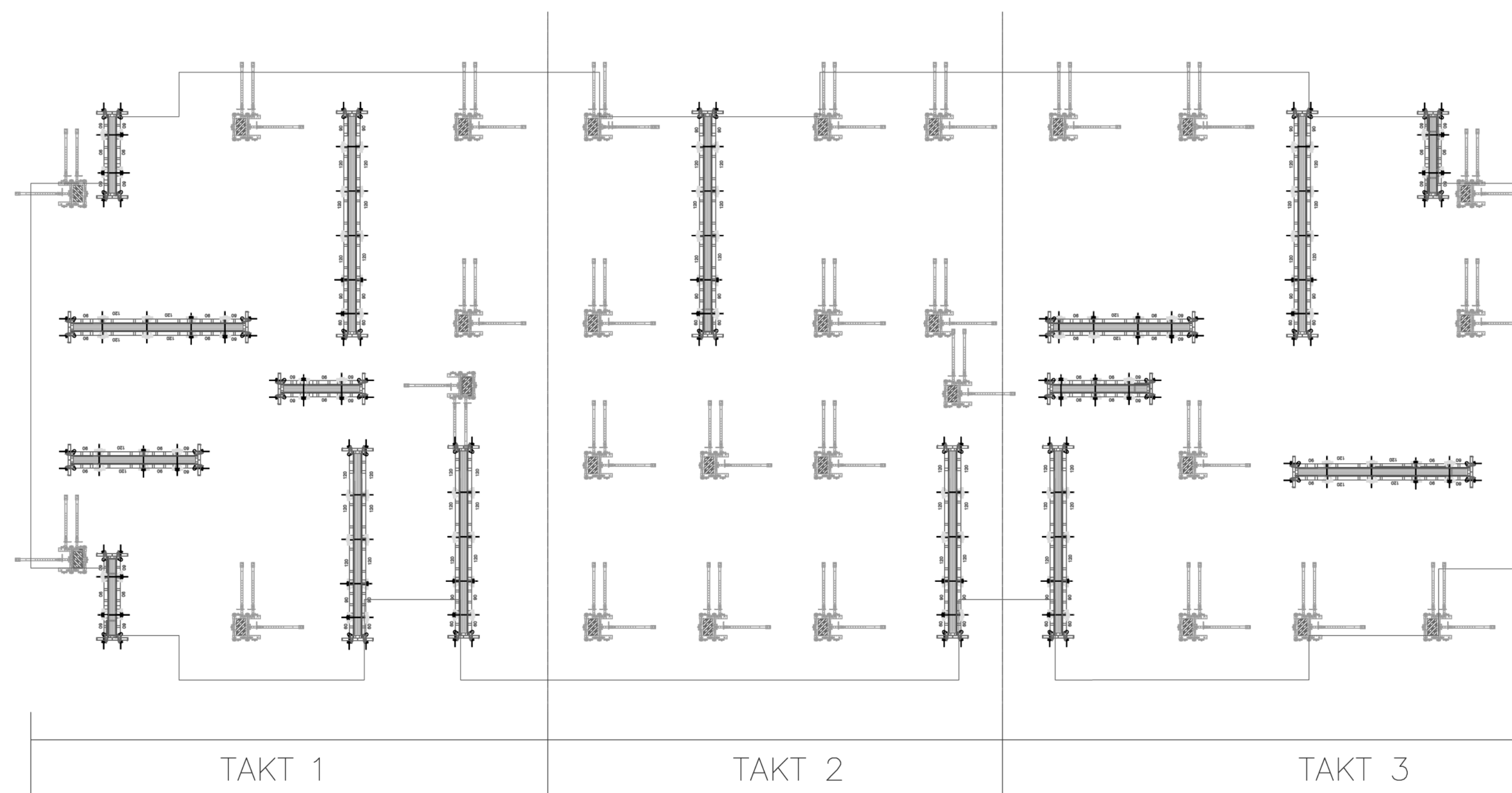
ТАКТ ПЛАН НА ХОРИЗОНТАЛНИ НОСЕЩИ ЕЛЕМЕНТИ – ПЛОЧА
