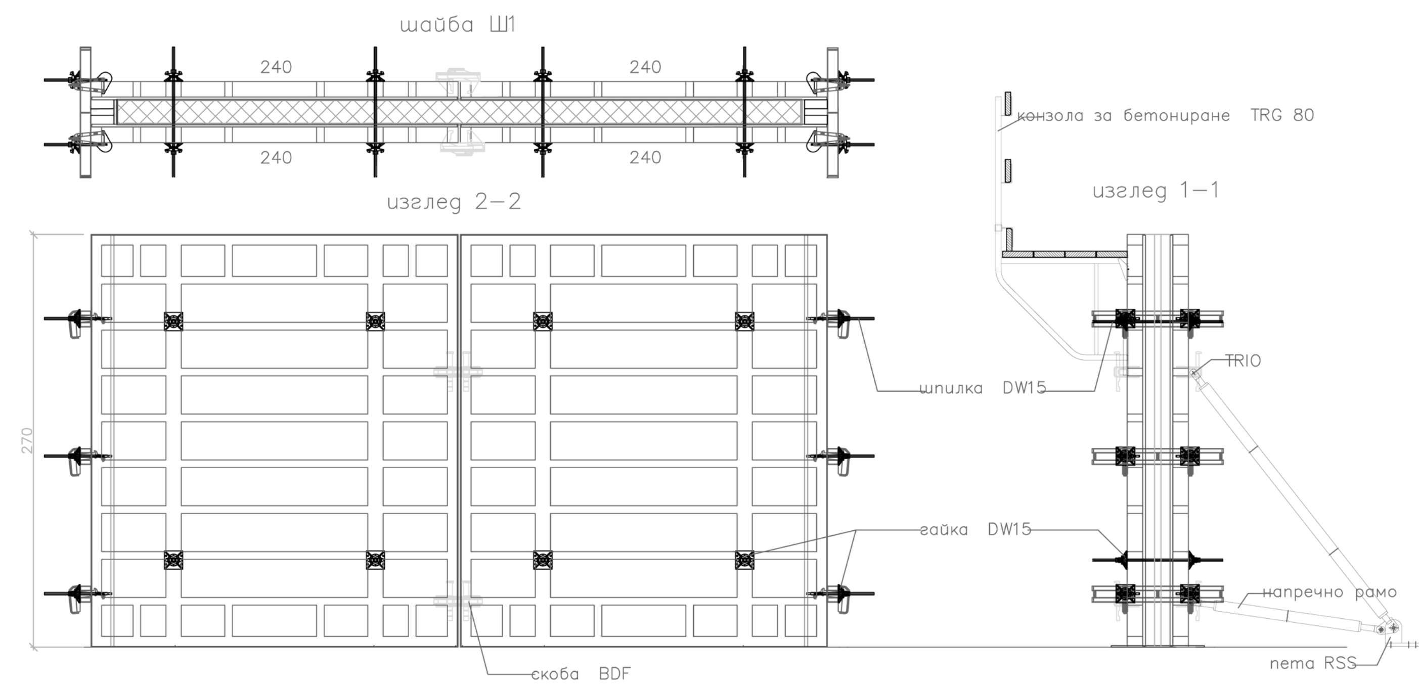
Детайл А
